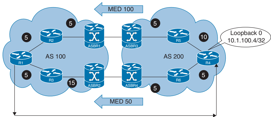
Figure 7-13 BGP Path Control Using MED Attribute
