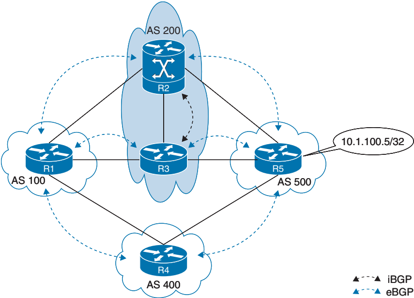
Figure 7-11 BGP MED Attribute
