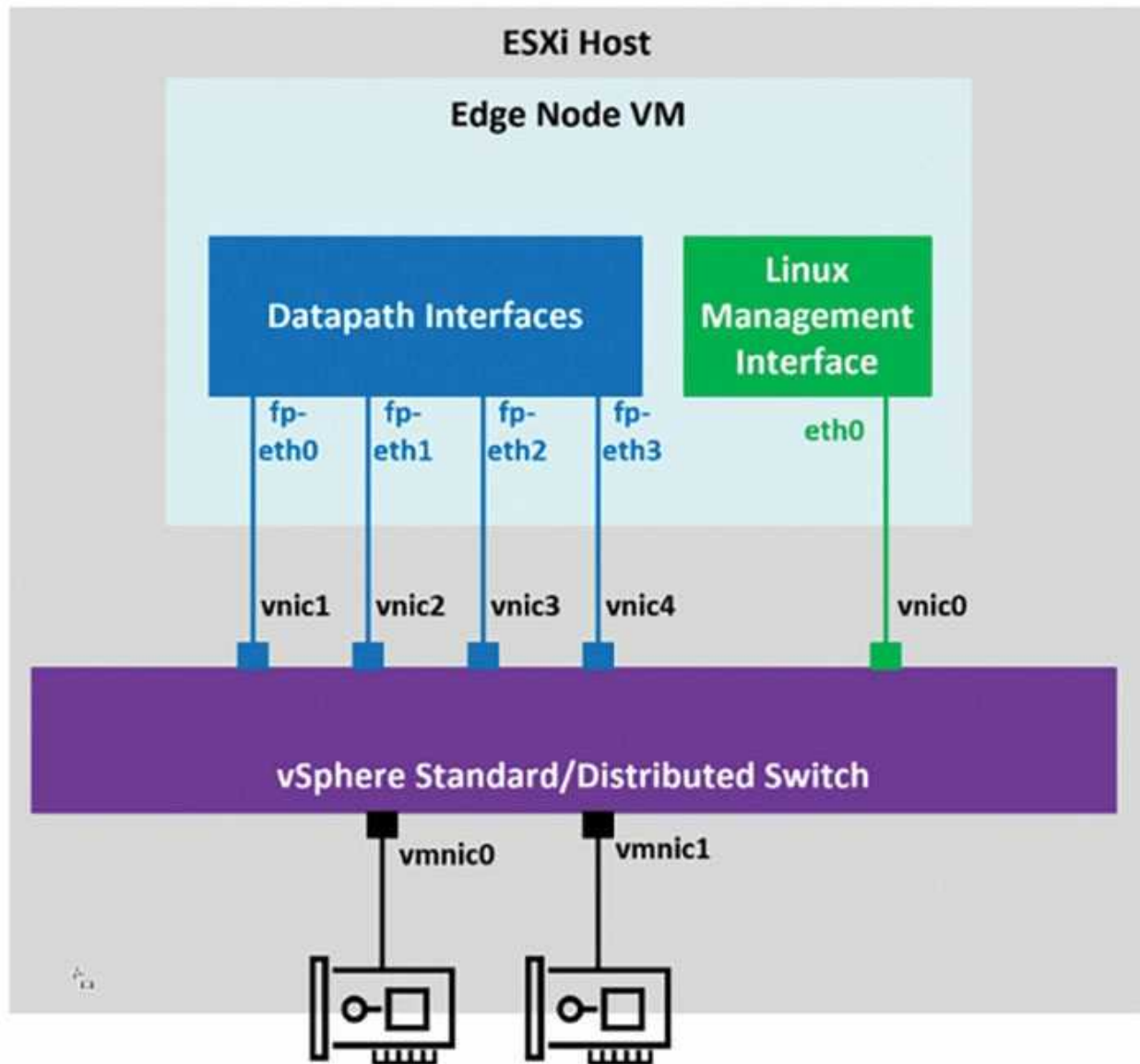
Figure 4.2: Edge VM interfaces
